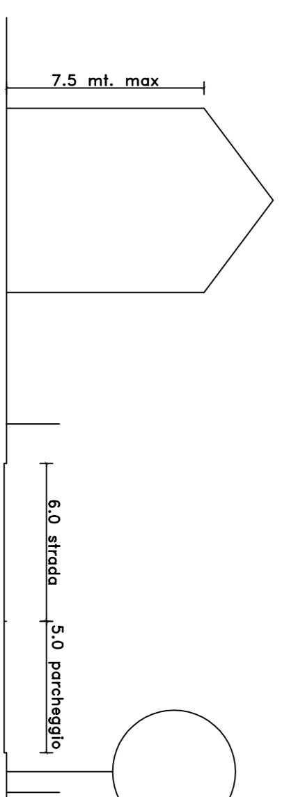
SEZIONE 2-2 Sc: 1:200
